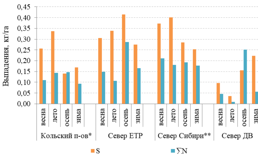
Рис. 4.40. Среднесезонные значения влажных выпадений серы (S) и суммарного азота (ΣN) в 2017 г. Примечание: без учета данных наблюдений за ХСО станций Мурманск и Никель*, Диксон, Норильск и Кюсюр**
