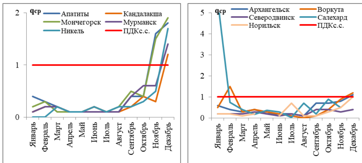
Рис. 4.46. Годовой ход бенз(а)пирена в городах АЗРФ в 2017 г., qcp, нг/м 3
