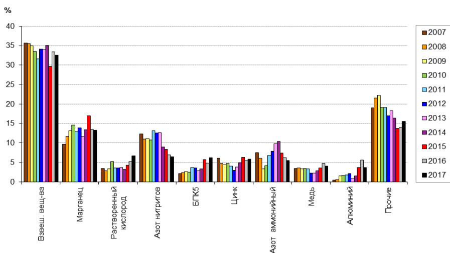
Рис. 3.52. Распределение случаев ВЗ и ЭВЗ поверхностных пресных вод по ингредиентам (в % от общего количества случаев ВЗ и ЭВЗ на территории Российской Федерации)
