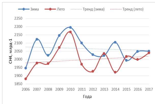
Рис. 2.17. Многолетние изменения средних сезонных концентраций CH 4 в приземном слое атмосферы на СКФМ в Приокско-Террасном биосферном заповеднике
