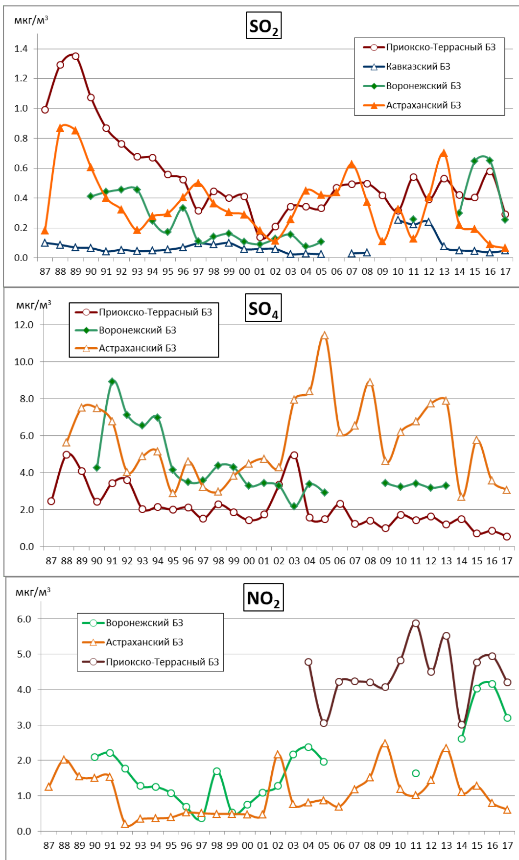
Рис. 2.16. Изменение фонового содержания диоксида серы, сульфатов и диоксида азота в атмосферном воздухе фоновых районов (мкг/м³)
