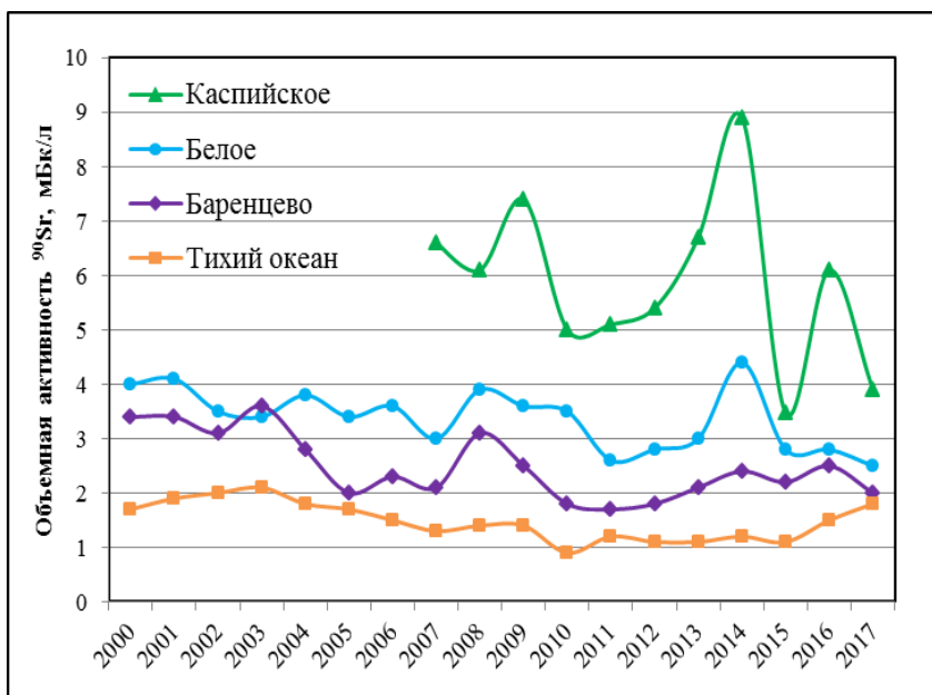
Рис. 4.59. Динамика объемной активности 90 Sr в прибрежных водах Белого и Баренцева морей в сравнении с водами Каспийского моря и Тихого океана вблизи восточного побережья Камчатки в 2000-2017 гг., мБк/л
