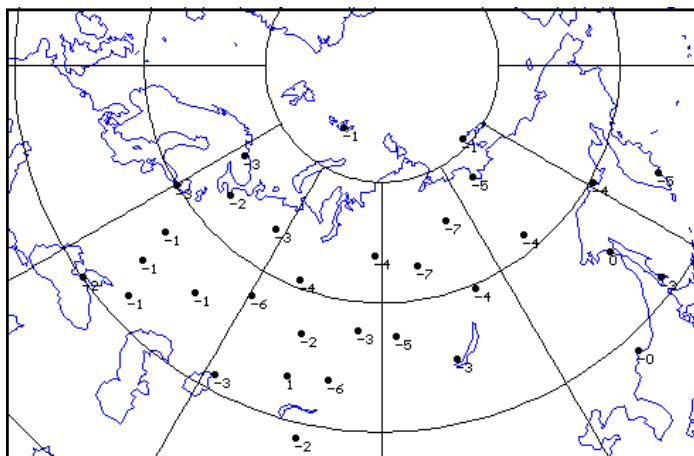
Рис. 2.9. Поле отклонений (%) общего содержания озона в 2017 г. от средних многолетних значений по данным озонометрической сети СНГ
