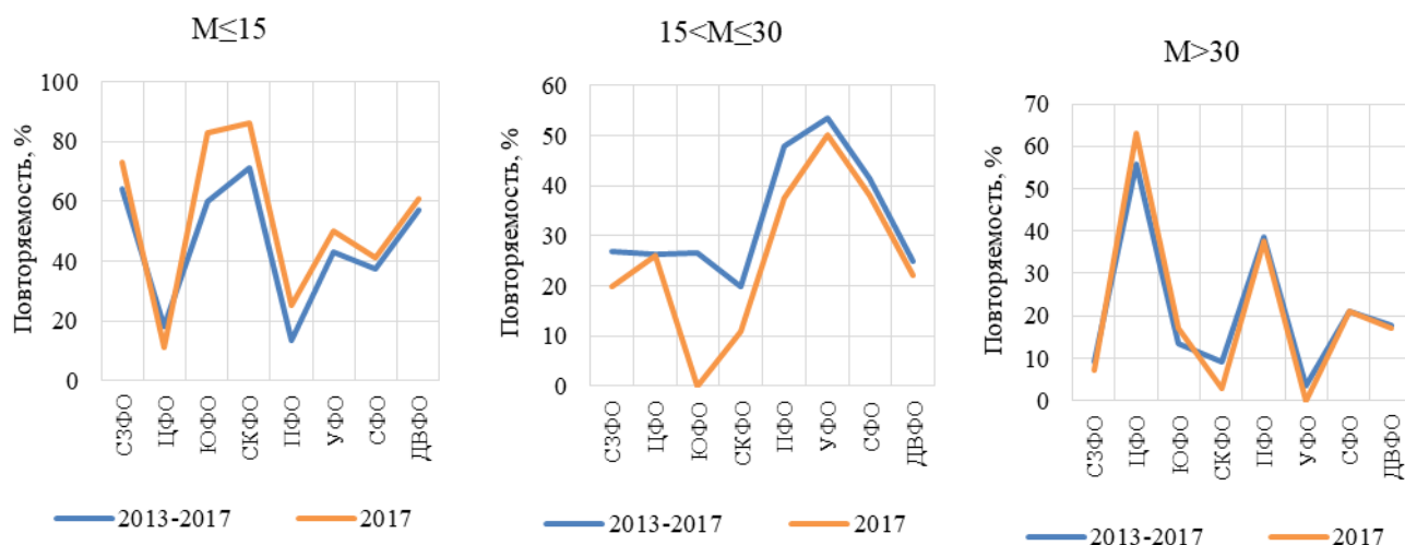
Рис. 2.23. Повторяемость (%) минерализации осадков (M, мг/л) по диапазонам в период с 2013 по 2017 гг.
