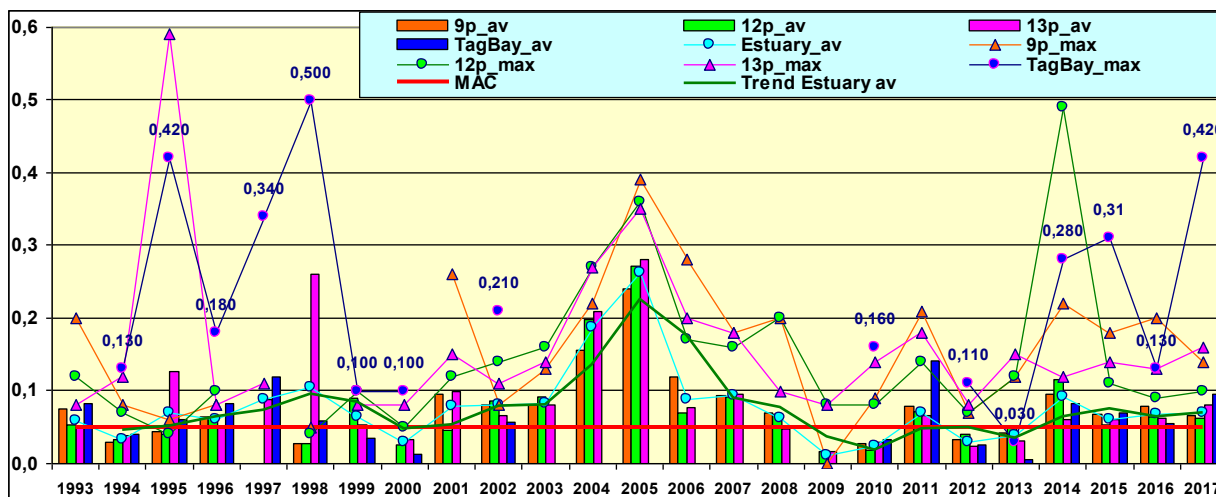
Рис. 3.55. Динамика средней и максимальной концентраций нефтяных углеводородов (мг/дм 3 ) в протоках дельты реки Дон и Таганрогском заливе в 1993-2017 гг. Примечание: 9р_av - средняя концентрация НУ на станции 9р; 9р_max - максимальная концентрация НУ на станции 9р; TagBay_av - средняя концентрация НУ в водах Таганрогского залива; Estuary_av - средняя концентрация НУ в водах русловых протоков Дона; MAC - ПДК; Trend Estuary av - тренд усредненной концентрации НУ в русловых протоках.
