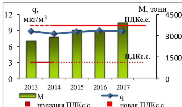
Рис. 3.14. Среднегодовые концентрации формальдегида (q, мкг/м³), величины санитарно-гигиенического норматива, ПДКс.с., мг/м³, выбросы от стационарных источников (M, тонн)
