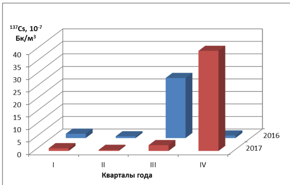
Рис. 4.57. Динамика средней за квартал величины объемной активности 137 Cs в воздухе г. Мурманск в 2016-2017 гг.
