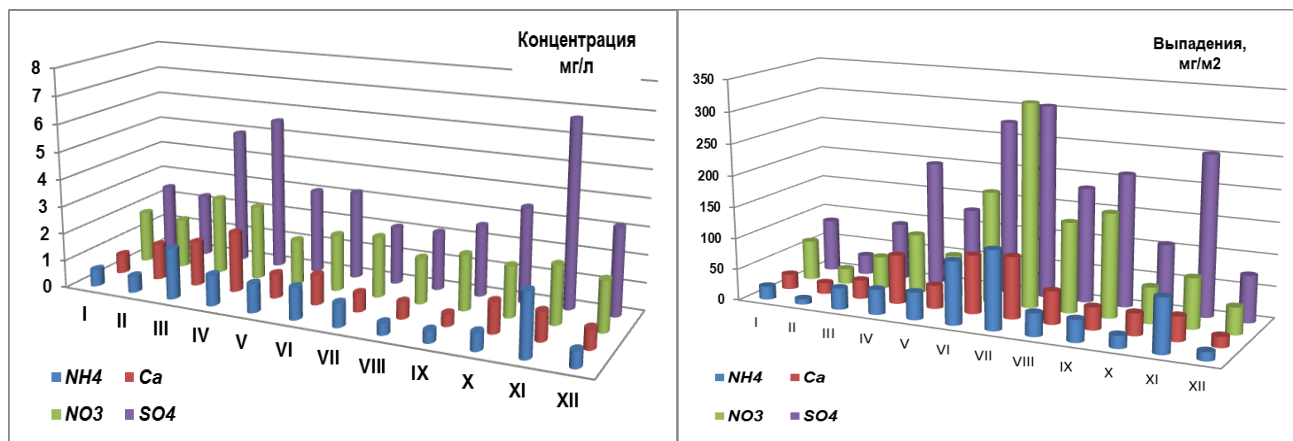
Рис. 2.35. Годовой ход концентраций (слева) и выпадений (справа) основных кислотообразующих ионов с осадками на Дальнем Востоке (ст. Приморская) в 2017 году
