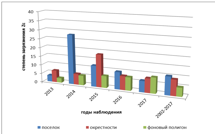
Рис. 4.61. Межгоддовая изменчивость суммарного показателя химического загрязнения Zс в районе пос. Баренцбург, его окрестностях и фоновых территориях в период 2013-2017 гг. и средние значения за 2002-2017 гг.
