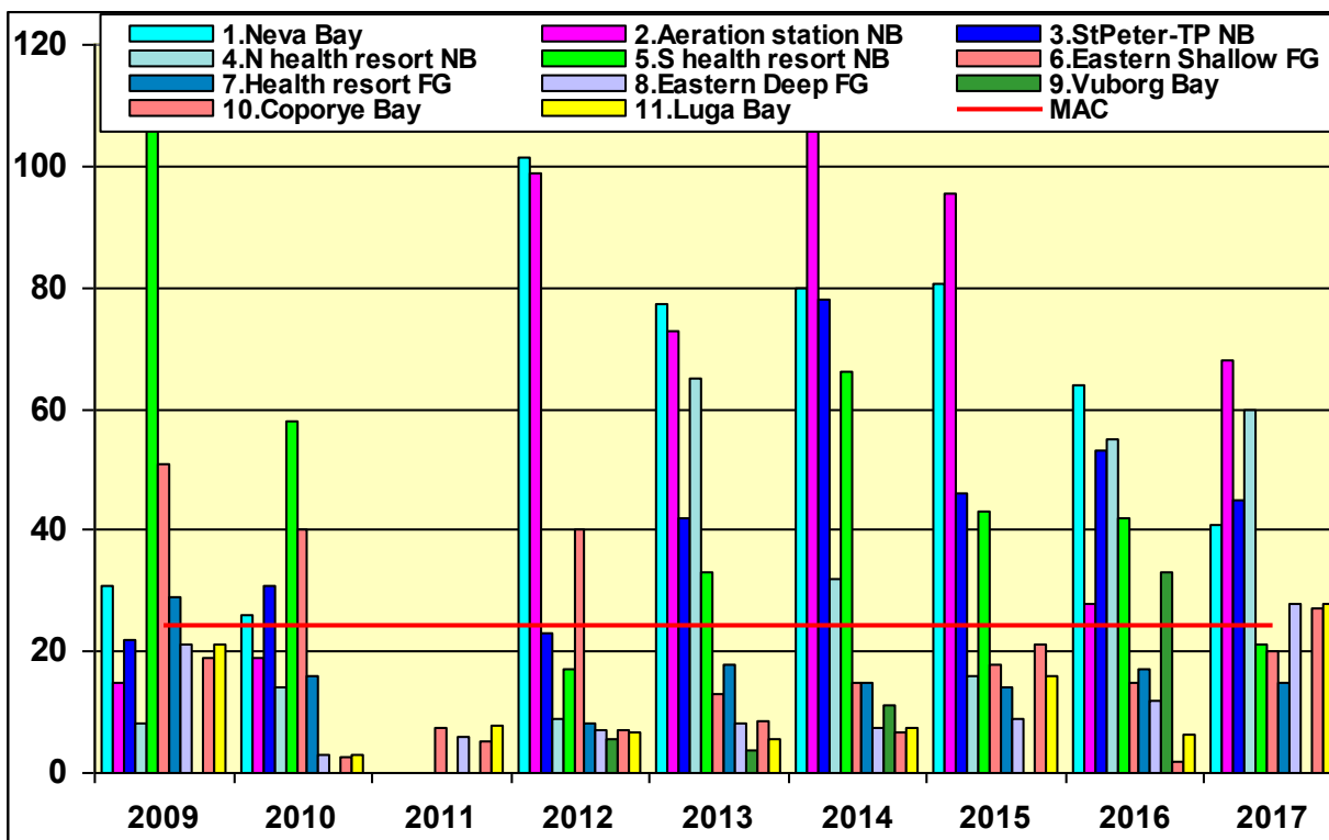
Рис. 3.60. Максимальная концентрация нитритного азота ( \text{мг}/\text{дм}^3 ) на различных участках акватории Невской губы и в восточной части Финского залива в 2009-2017 гг.
