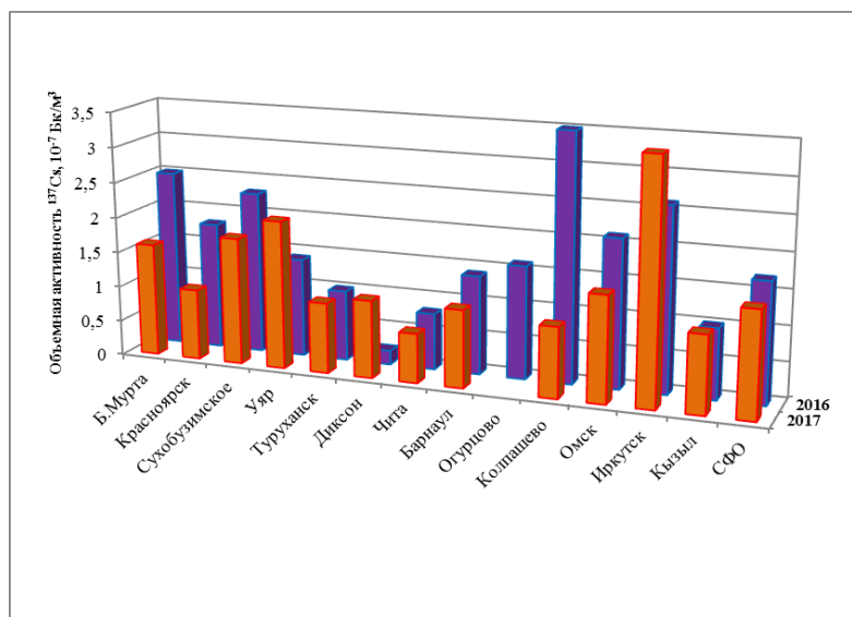
Рис. 2.40. Среднегодовая объемная активность 137 Cs в населенных пунктах СФО в 2016-2017 годах, 10 -7 Бк/м 3
