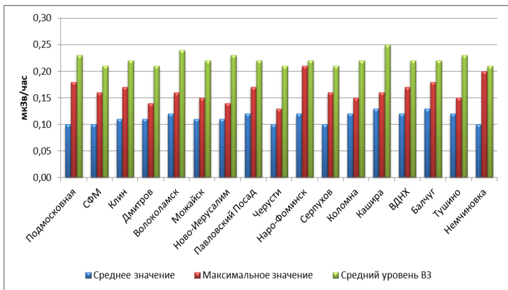
Рис. 4.15. Мощности AMBIENTного эквивалента дозы (МАЭД) на станциях Московского региона в 2017 году
