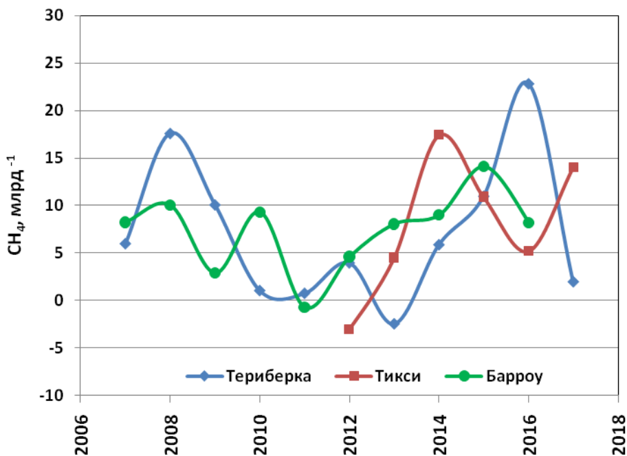
Рис. 2.2. Межгодовые изменения концентрации \text{CH}_4
