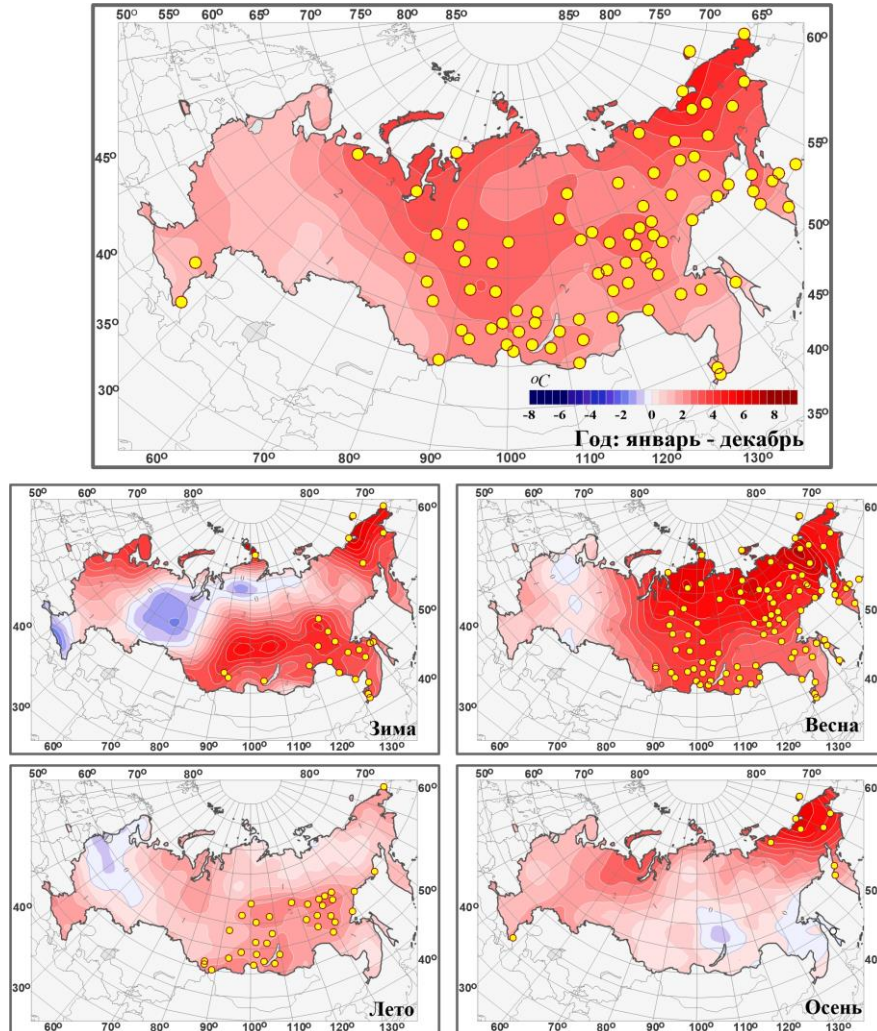
Рис. 1.9. Аномалии средней годовой и сезонных температур приземного воздуха на территории России в 2017 г. (отклонения от средних за 1961-1990 гг.) с указанием локализации экстремальных аномалий. Кружками белого и желтого цвета показаны станции, на которых наблюденная температура оказалась ниже 5-го или выше 95-го процентиля.
