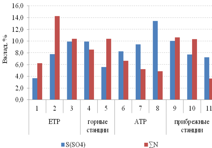
Рис. 2.22. Вклад серы и азота в структуру суммарных влажных выпадений, 2017 г. 1 - Усть-Вымь, 2 - Приокско-Тerrasный БЗ, 3 - Воронежский БЗ, 4 - Кавказский БЗ, 5 - Шаджатмаз, 6 - Памятная, 7 - Туруханск, 8 - Хужир, 9 - Приморская, 10 - Терней, 11 - Тикси
