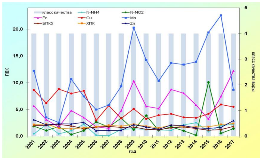
Рис. 3.26. Изменение среднегодовых концентраций отдельных ингредиентов и качества воды р. Охта,
