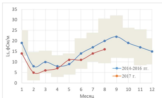
Рис. 4.33. Годовой ход L_5 в 2017 2 мая 2014 г. N 287 на фоне осредненного годового хода L_5 за период 2014-2016 гг. Цветным фоном обозначены границы стандартного отклонения от среднего значения за 2014-2016 гг.
