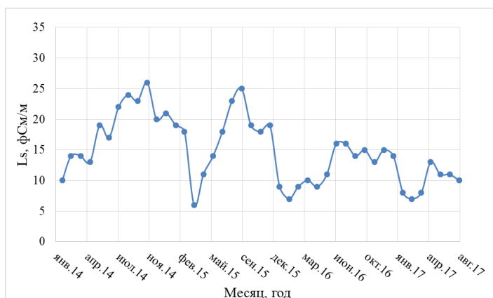
Рис. 4.31. Среднемесячные значения L_5 по данным наблюдения на ГМО Тикси в период 2014-2017 гг.
