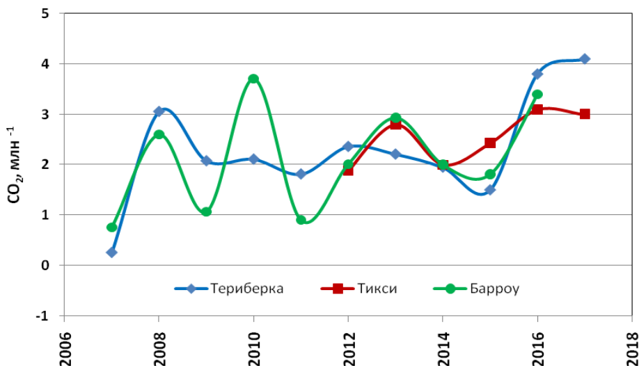
Рис. 2.1. Межгодовые изменения концентрации \text{CO}_2
