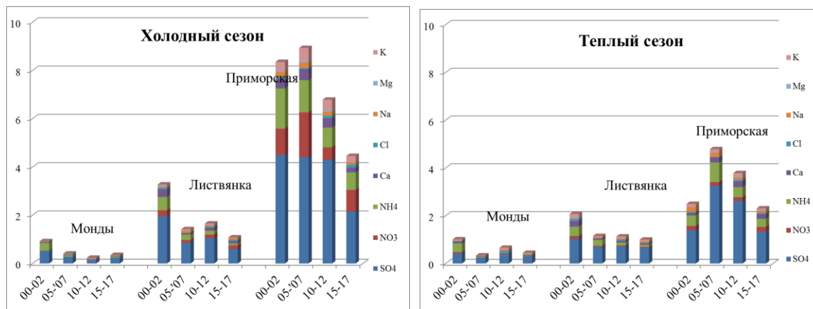
Рис. 2.33. Изменение среднего химического состава аэрозолей (мкг/м 3 ) на станциях ЕАНЕТ в холодный (слева) и теплый (справа) периоды по наблюдениям в 2000-2017 г.
