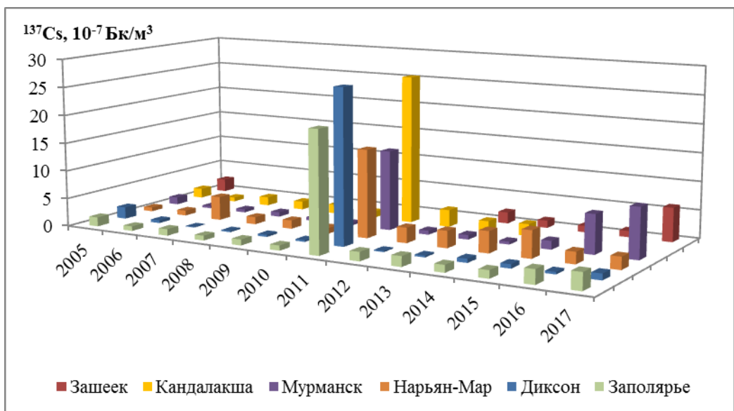
Рис. 4.56. Объемная активность 137 Cs в приземной атмосфере в пунктах наблюдения Сухопутных территорий Арктики и в среднем по Заполярью в 2005-2017 гг., 10 -7 Бк/м 3
