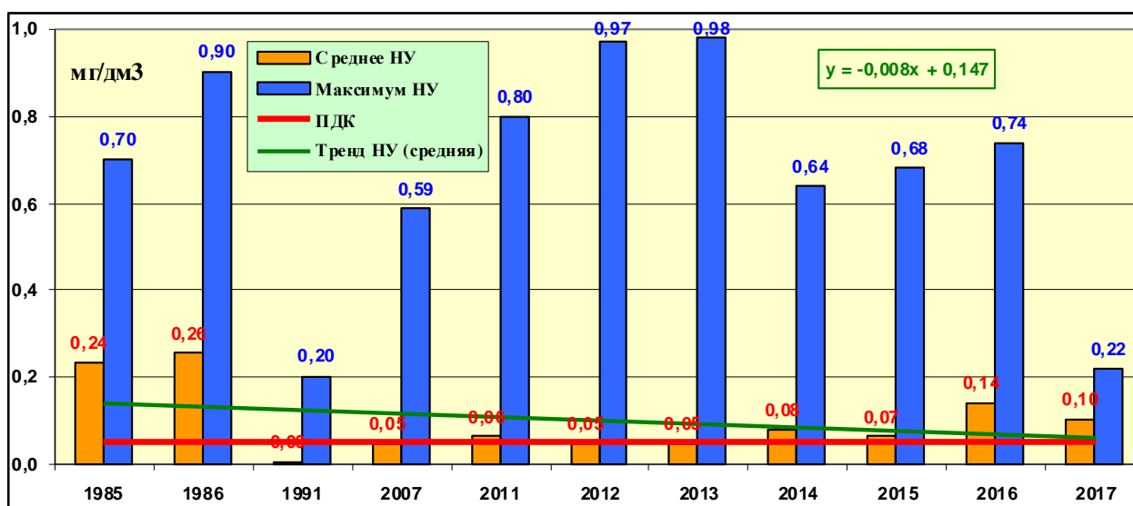
Рис. 3.62. Динамика средней и максимальной концентраций нефтяных углеводородов (мг/дм 3 ) в водах Авачинской губы на Камчатке в 1985-2017 гг.
