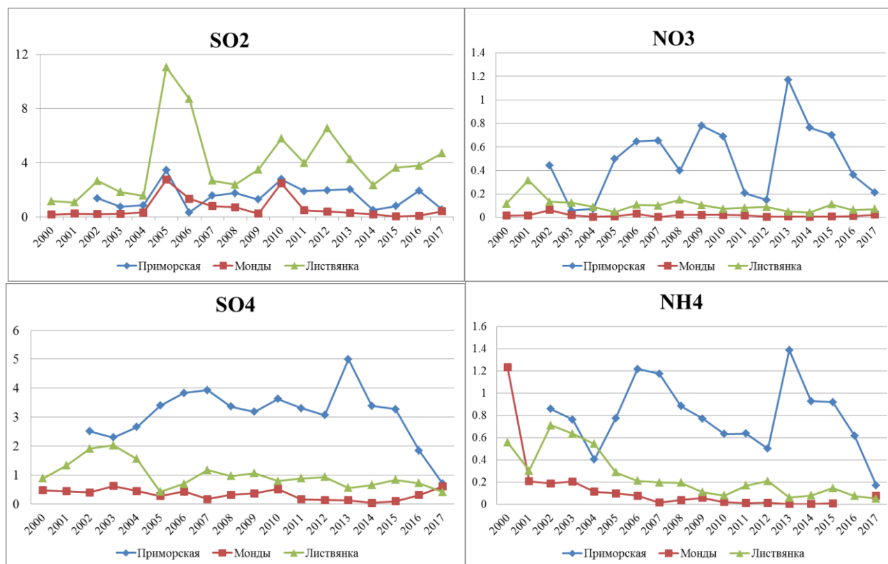
Рис. 2.34. Изменения средних годовых концентрации соединений серы (слева) и азота (справа) в воздухе на станциях ЕАНЕТ (мкг/м 3 )
