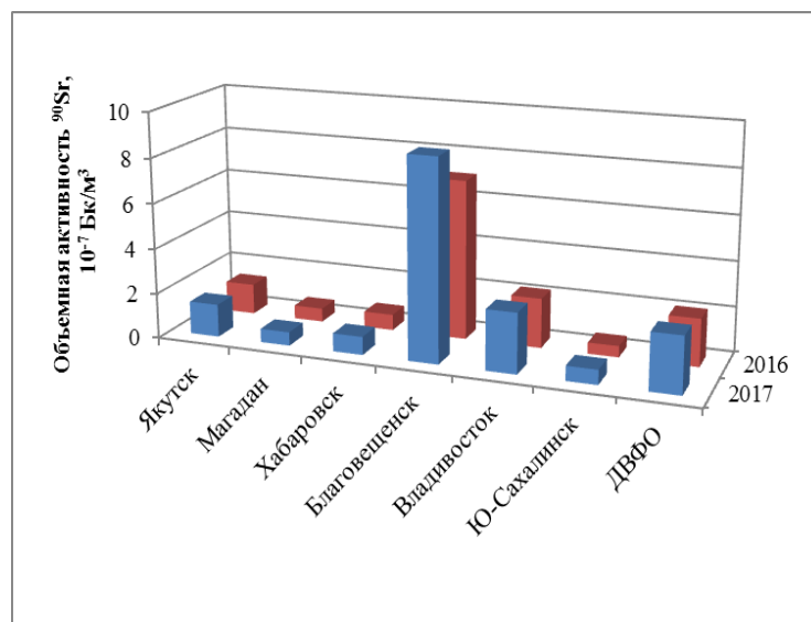
Рис. 2.41. Среднегодовая объемная активность 90 Sr в населенных пунктах ДВФО в 2016-2017 годах, 10 -7 Бк/м 3
