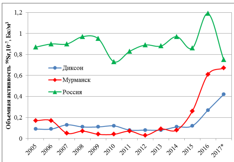
Рис. 4.58. Динамика объемной активности 90 Sr в воздухе на о. Диксон, в г. Мурманск и средневзвешенной по России в 2005-2017 гг. (в 2017 г. данные за первое полугодие)
